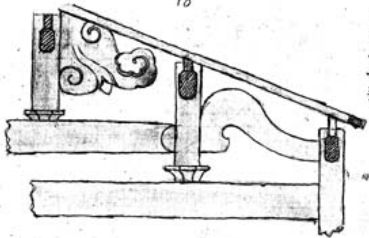
海老虹梁ノ用法ヲ見ル頗ル奇き。
