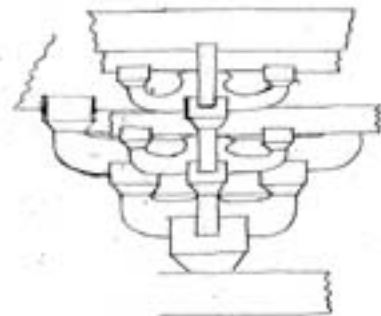
斗様新圖
