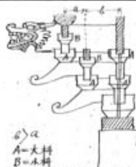
斗拱断面
