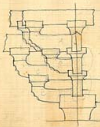
○塔八角七重 光緒蘇州北寺塔の図
