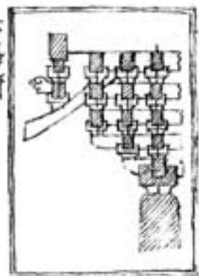
下層軒
