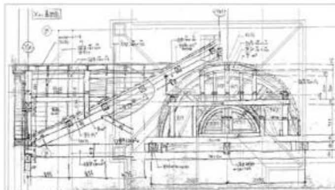
ドーマー部スケッチ
