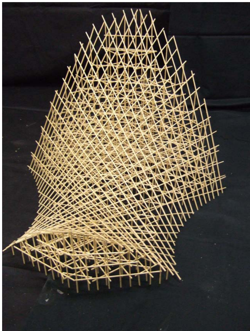
図 型枠のためのフレーム模型
