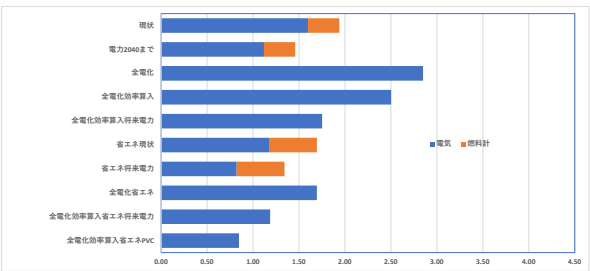
図 3 戸建集合平均 tCO 2 /年度 電力・燃料別
